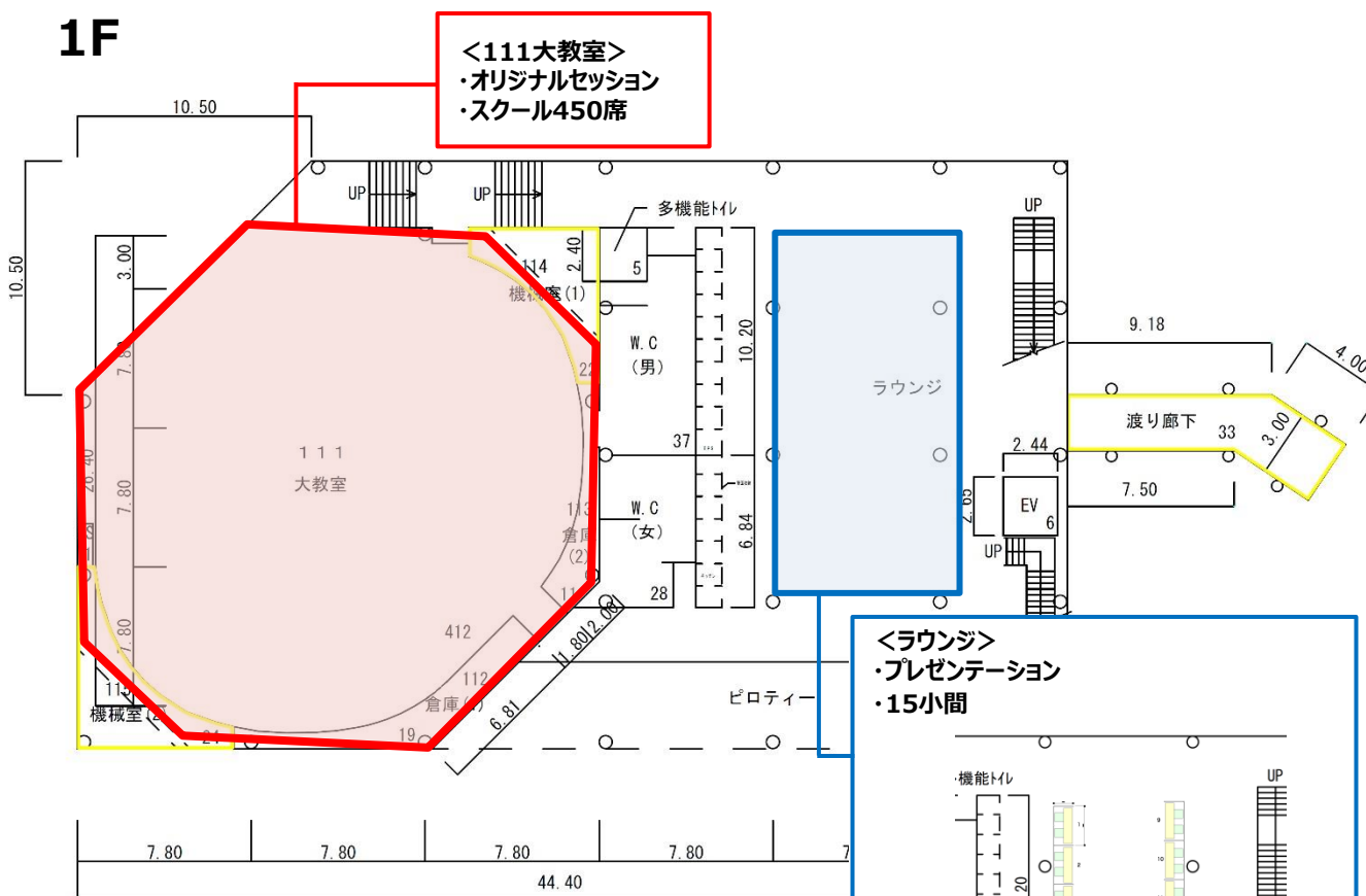
1階平面図 S = 1 : 400
