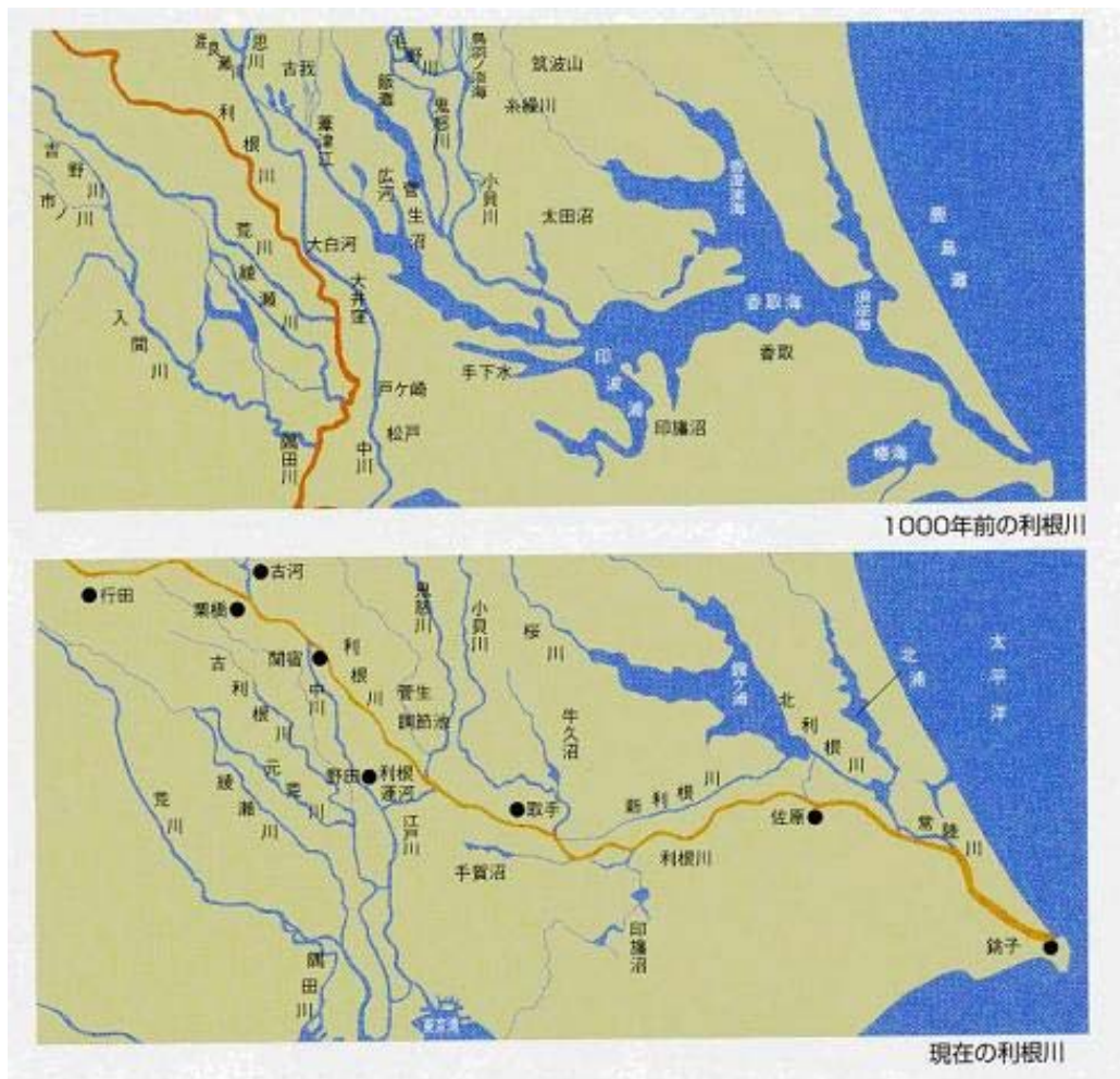
図 1-1 昔と今の利根川流域（国土交通省利根川上流河川事務所提供）
