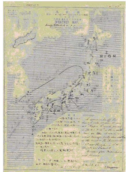
図 6-2 1890年9月16日の天気図 高知県沖に台風が接近している(気象庁提供)
