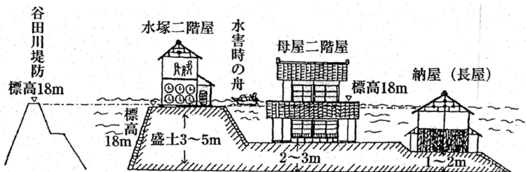
図 1-5 板倉町の水塚・母屋と堤防との相関図
