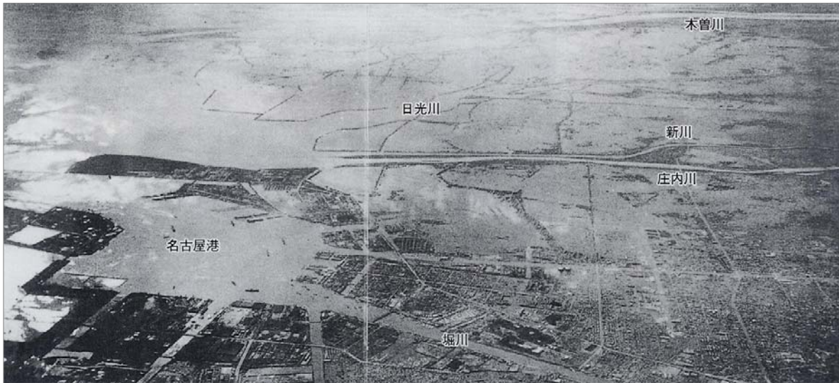
写真2-1 泥の海と化した伊勢湾奥の低平地の状況
