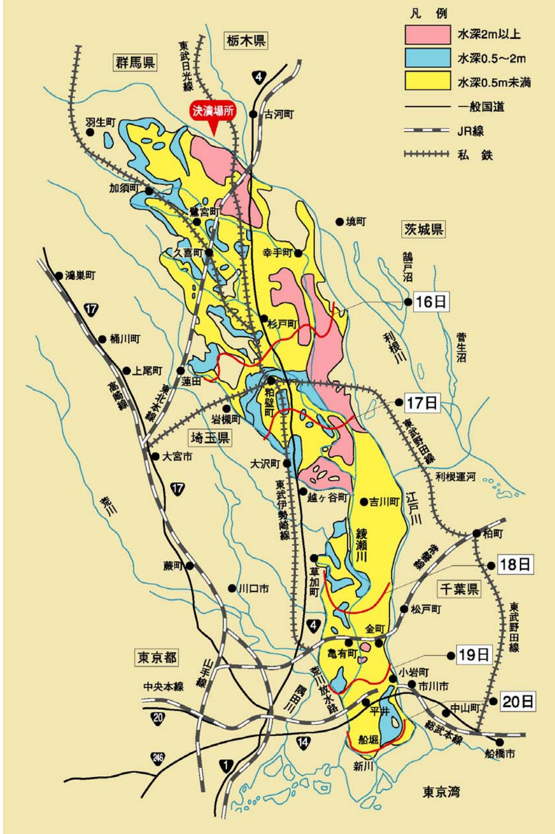
図1-4 カスリーン台風による利根川の氾濫流（浸水深と氾濫流の到達時間）
