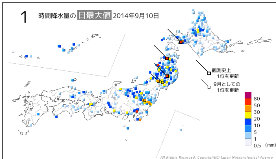
1時間降水量の日最大値(5mm以上のみ)
