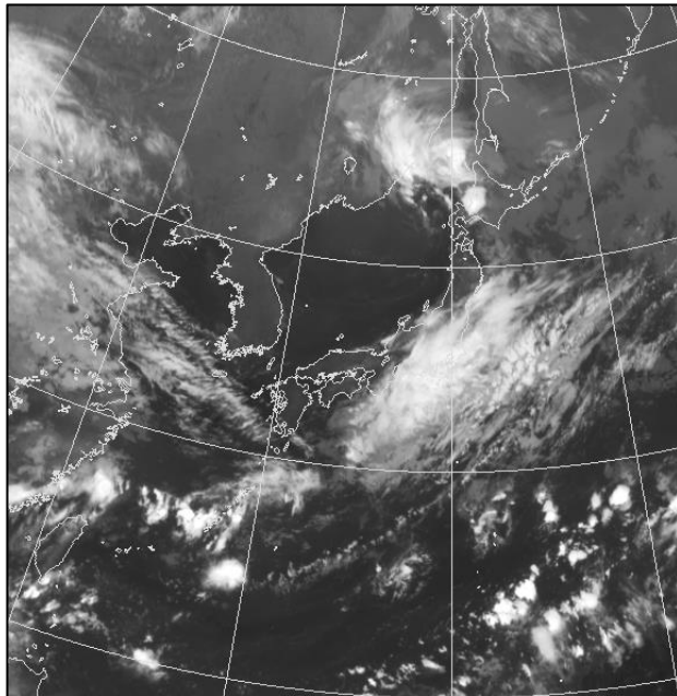
衛星画像(赤外) 9月11日6時
