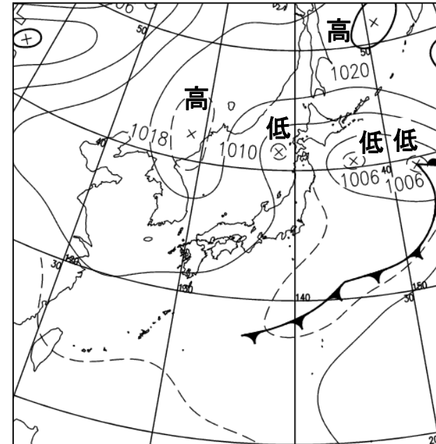
予想天気図 9月12日21時
