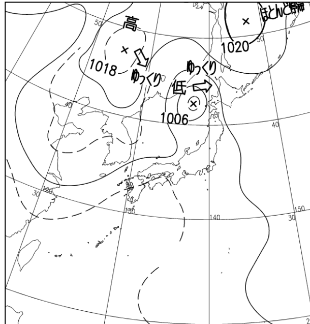
地上天気図 9月11日6時
