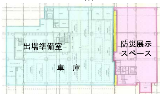
<1階>
